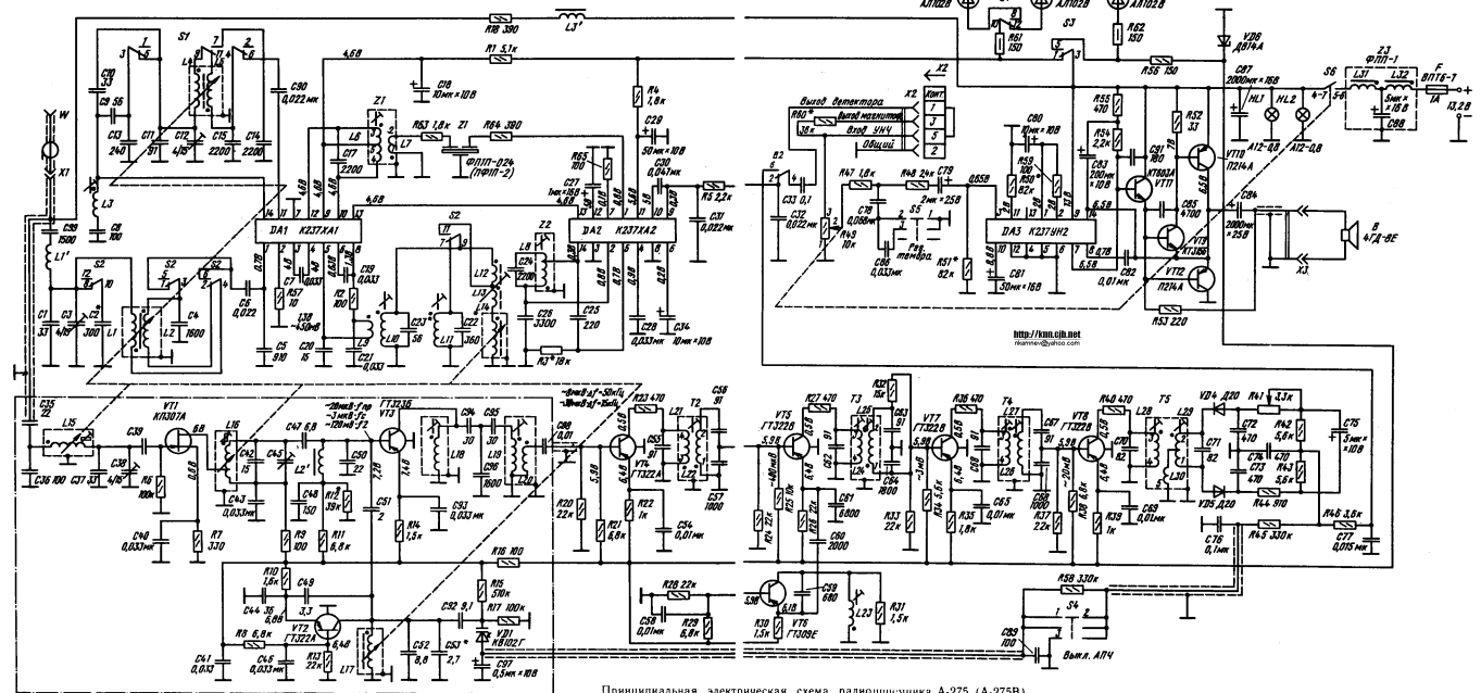
Принципиальная электрическая схема радиоприемника А-275 (А-275В)
