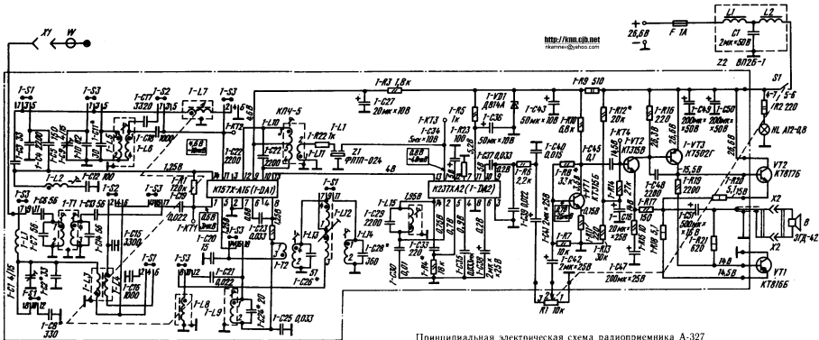
Принципиальная электрическая схема радиоприемника А-327
