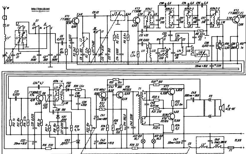
Принципиальная электрическая схема радиоприемника А-370 (А-370М, А-370М1)
