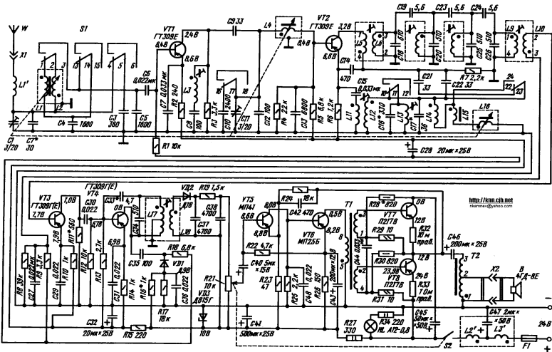
Принципиальная электрическая схема радиоприемника А-324
